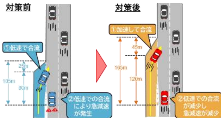
図－7 名阪国道の事故対策事例(久我IC オンランプ改良)
